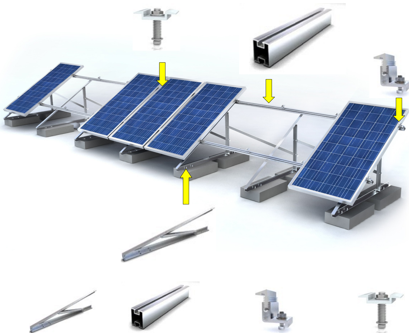
verstelbare driehoek
